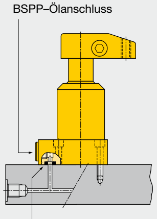
Integrierter O-Ring-Anschluss
