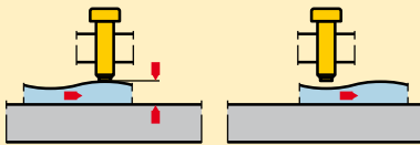
Abbildung 7 Starres Spannen
