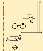
Turbo-Air-Hydraulikpumpe für CETOP03-Ventile Beispiel PASG-3002SB
