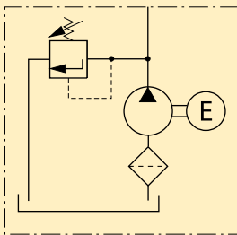
Einstufige elektrische Pumpe Beispiel ZW4010NE-S
