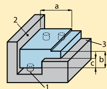
Abbildung 5a Werkstück mit Bestimmenebene
