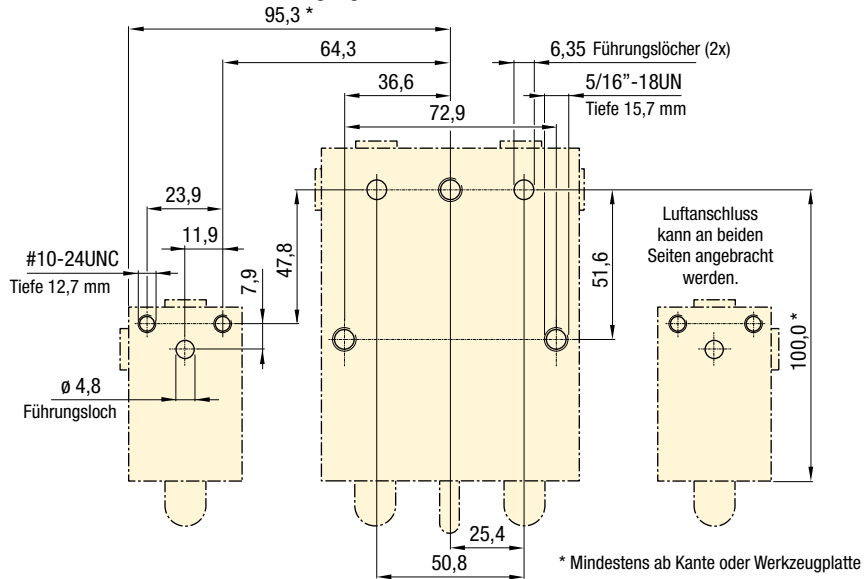
MCRC-21 mit MCRA-11 Palettenteil mit Luftanschluss und mit vorgesteuertem Rückschlagventil – Befestigungslochbild
