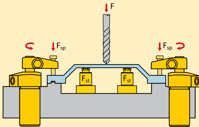
Abbildung 9 Abgestützte Werkstücke.
