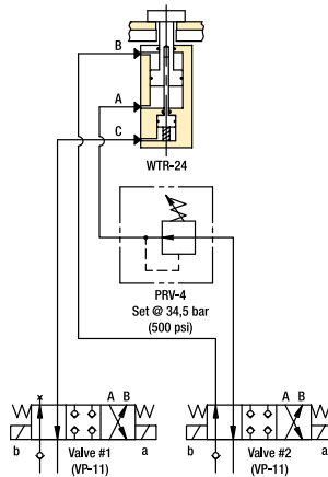
Flache Drehbewegung von -90°
