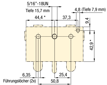
MCRC-21 mit MCRA-11 Palettenteil mit Luftanschluss und mit vorgesteuertem Rückschlagventil – Befestigungslochbild
