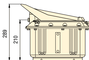
PATG-Serie
