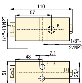
HV-1000A
