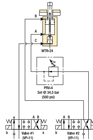
Flache Drehbewegung von -90°
