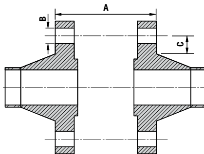
Flanschabmessungen
