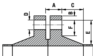
Flanschabmessungen
