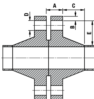
Flanschabmessungen
