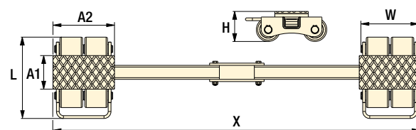
EMLSD-Serie, Doppelmitlaufwagen
